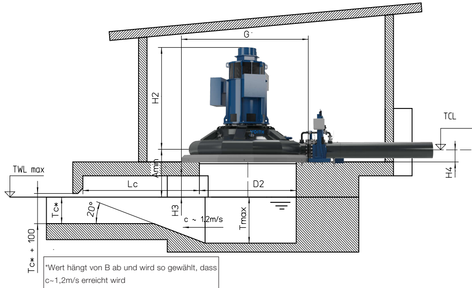
Schnittansicht A-A
